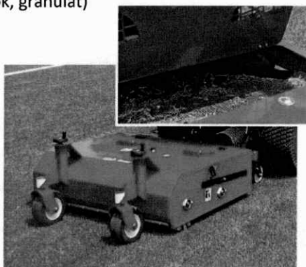
Kefy na údržbu umelých povrchov s výplňou (piesok, granulát)
