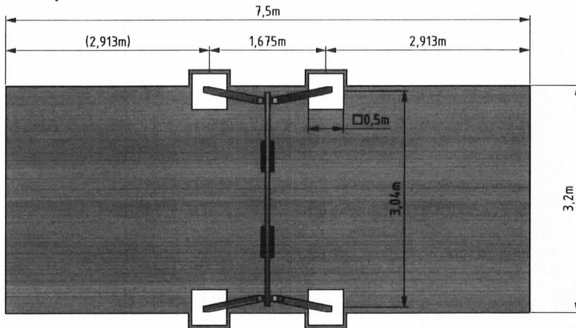
Technický náčrt
